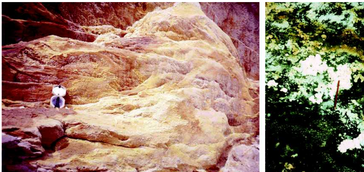
Figura 3.14 Ejemplos de Minerales Generadores de Acidez. Izquierda: en el Tajo de una Mina al Cielo Abierto de Oro, Ghana. Derecha: Aluminocopiapita (blanco) encima de Szomolnokita (turquesa) en una Galería Subterránea, Milluni, Bolivia.
