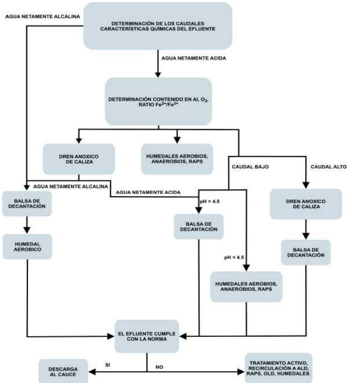
Figura 5.1 Esquema del diagrama de flujo para la Selección de Tratamientos Pasivos de Aguas Acidas. Basado en Younger et al, 2002 y Wolkersdorfer, 2006
